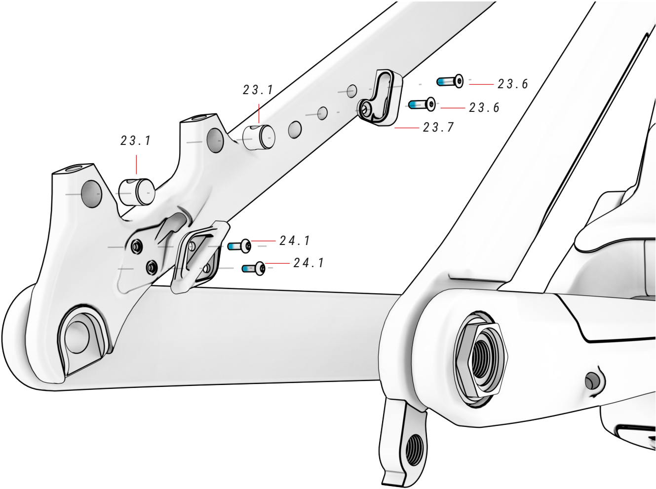
24 SNELHEIDSSENSORSCHROEF
