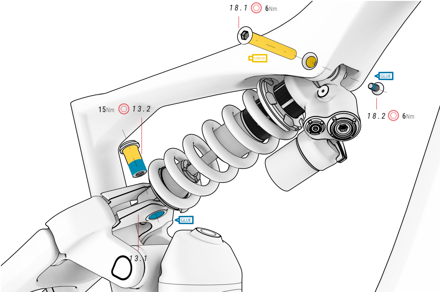
13 CLEVIS ref.: 381553900
