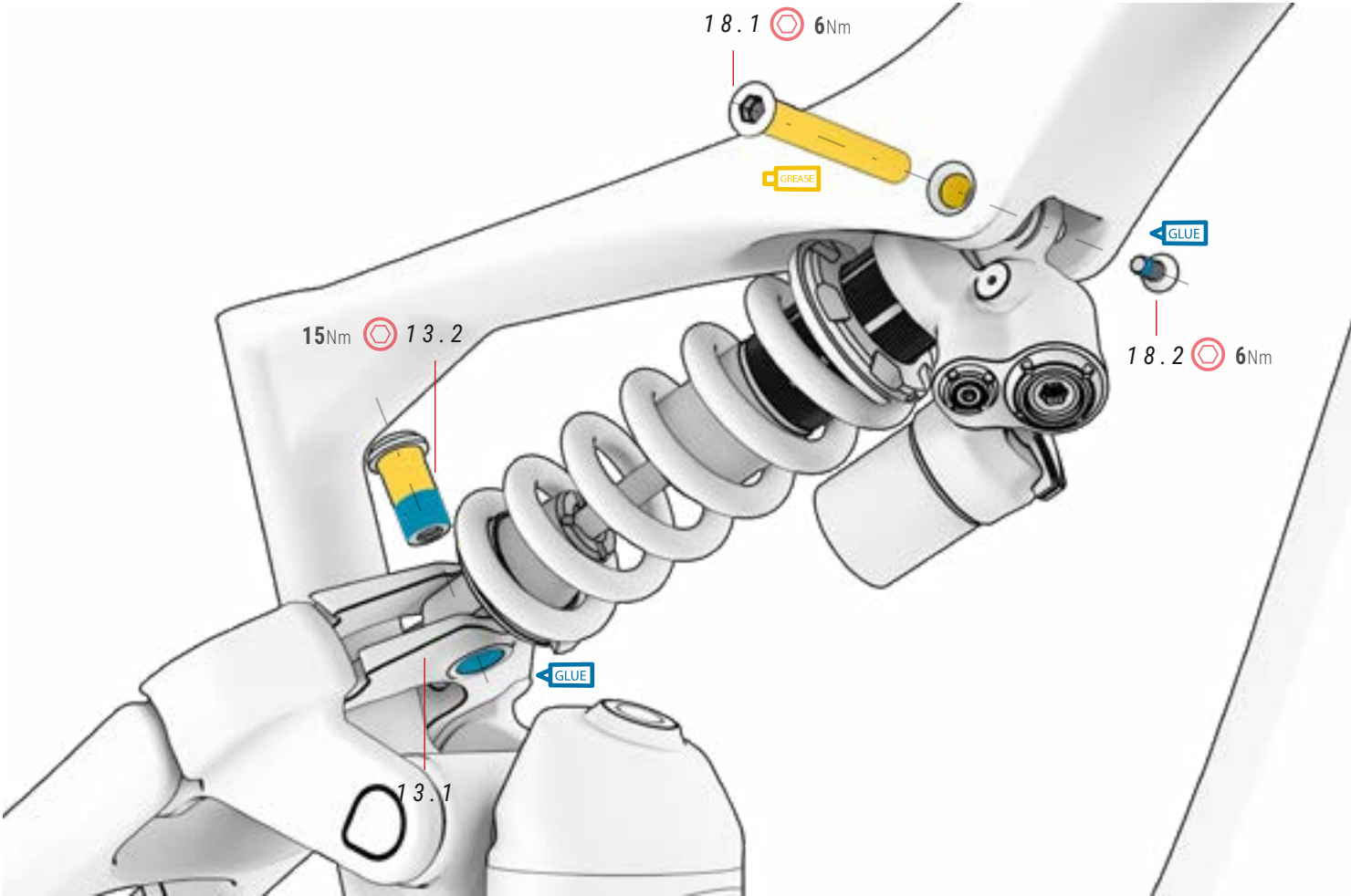
13 CLEVIS ref.: 391817500
