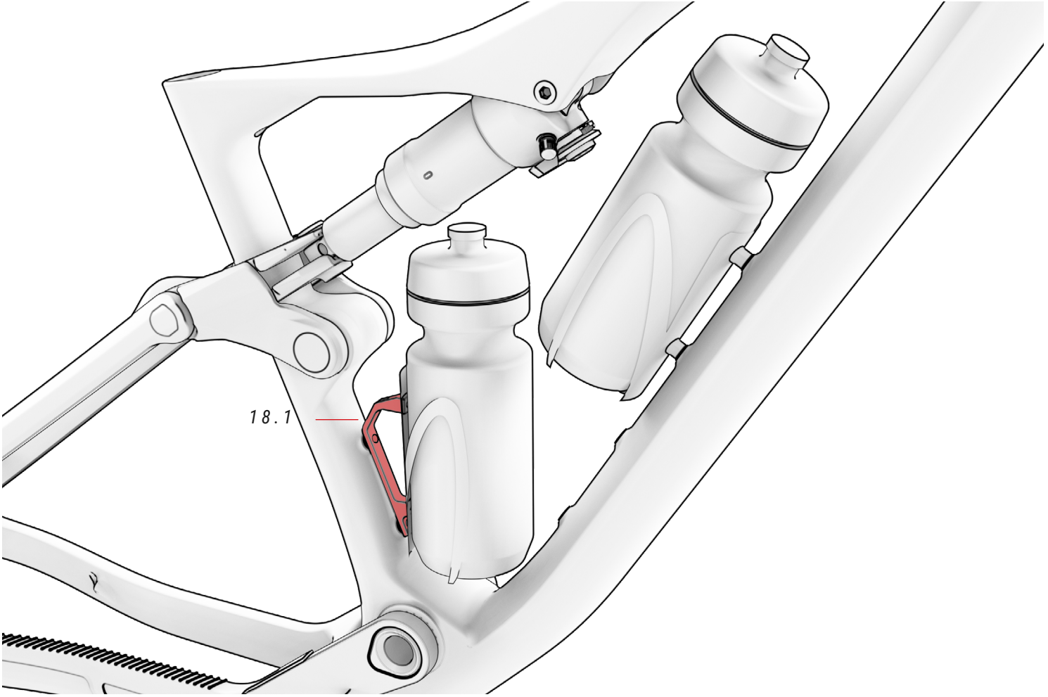
18 ADAPTATEUR DE BOUTEILLE ref.: 387461600
