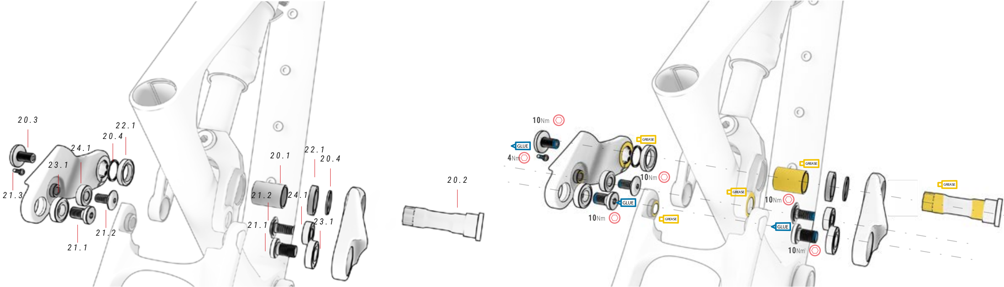
20 AXE E VIS DE BIELLE ref.: 391834800
