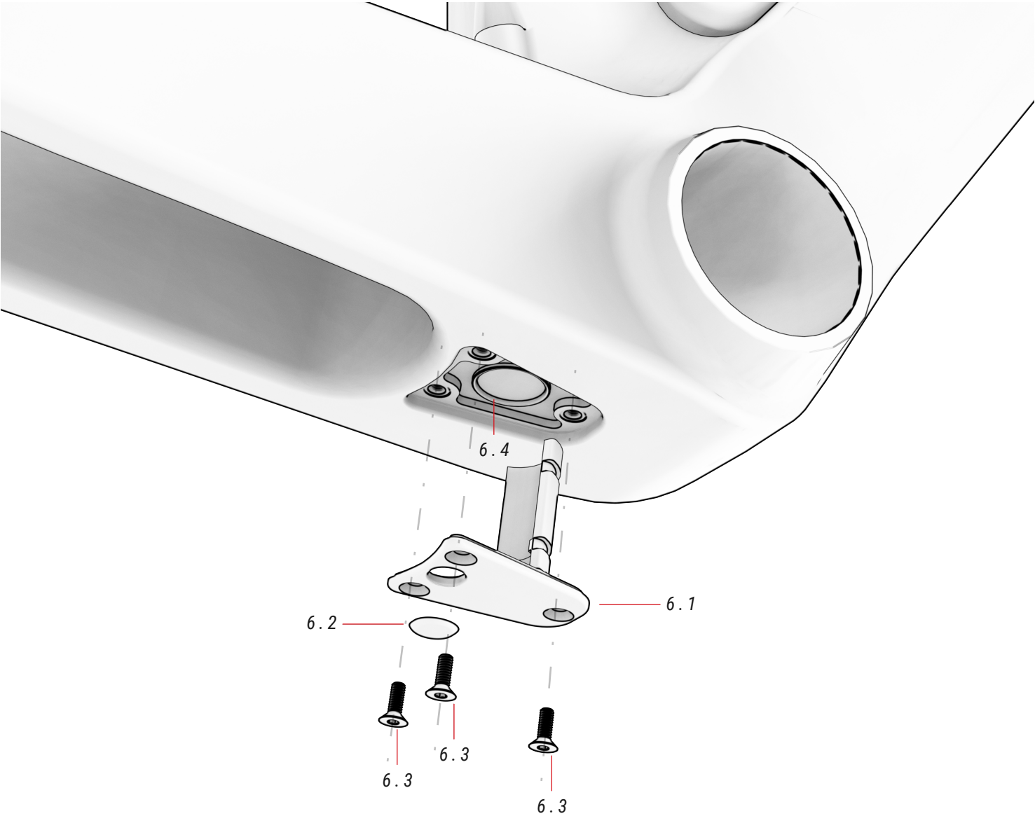
06 ALLOGGIAMENTO DELLA BATTERIA ref.: 381548100
