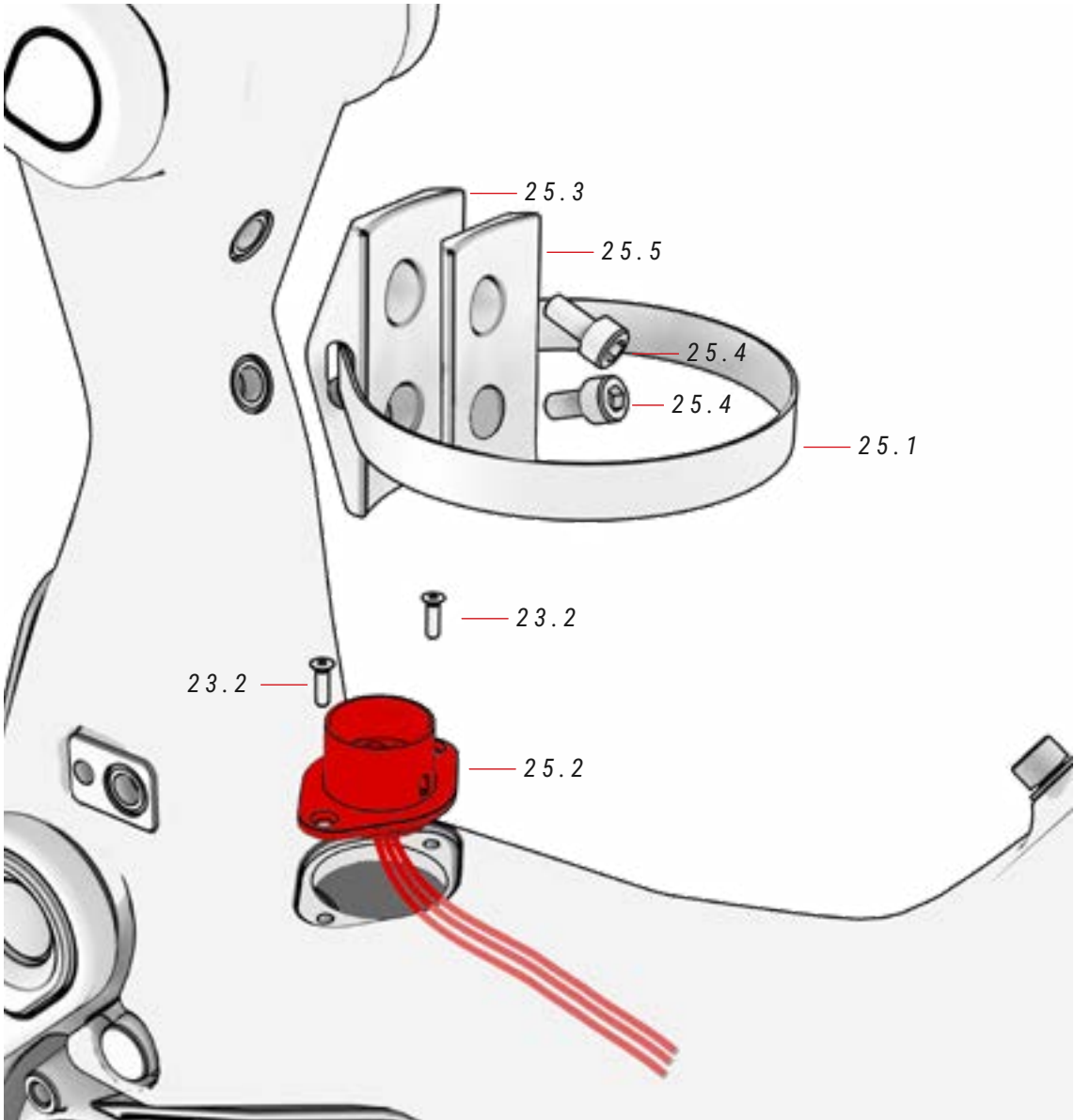
25 KIT BATTERIA XPRO DD ref.: 387481200
