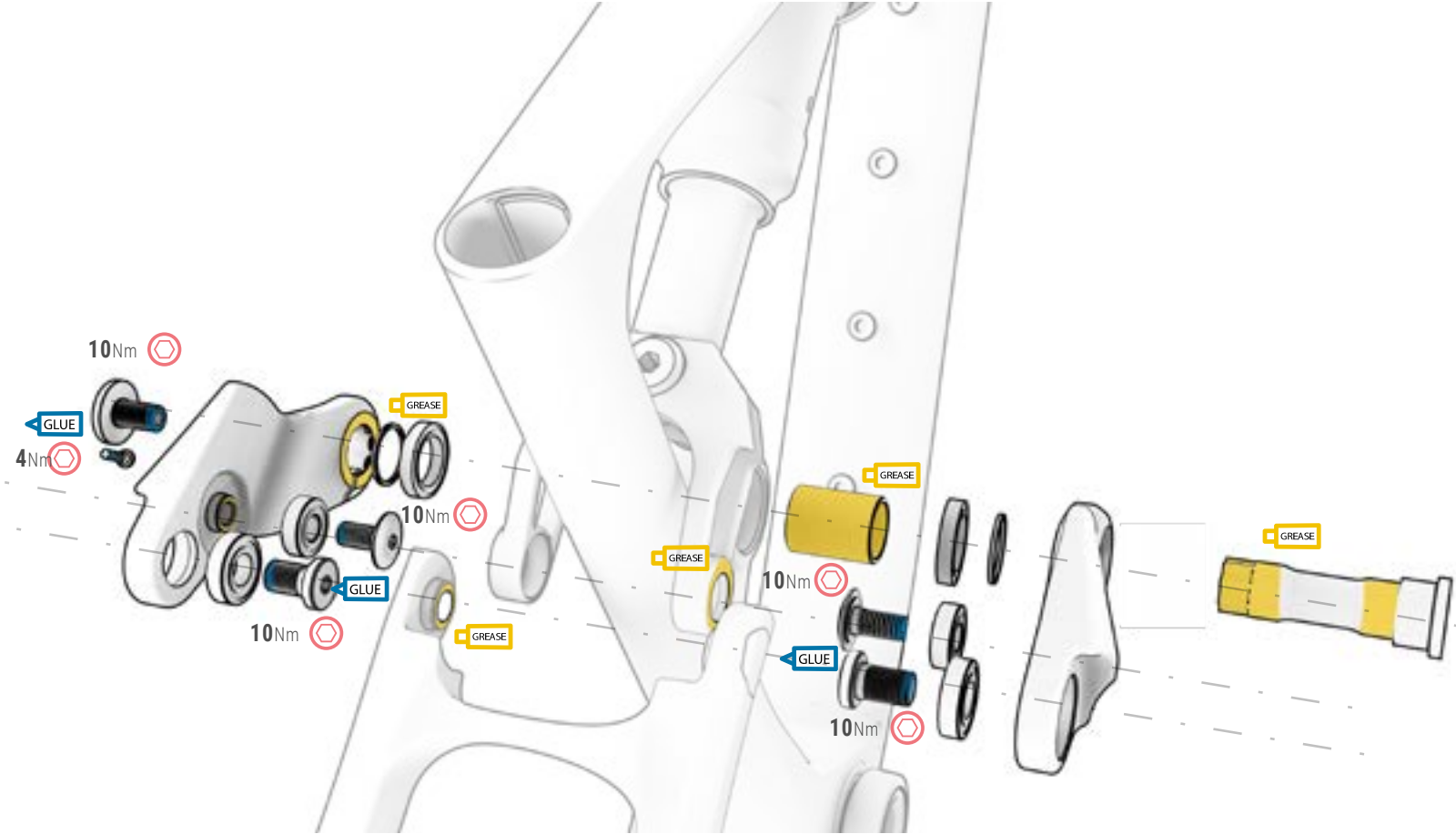
22 ROLAMENTO ref.: 391839800
