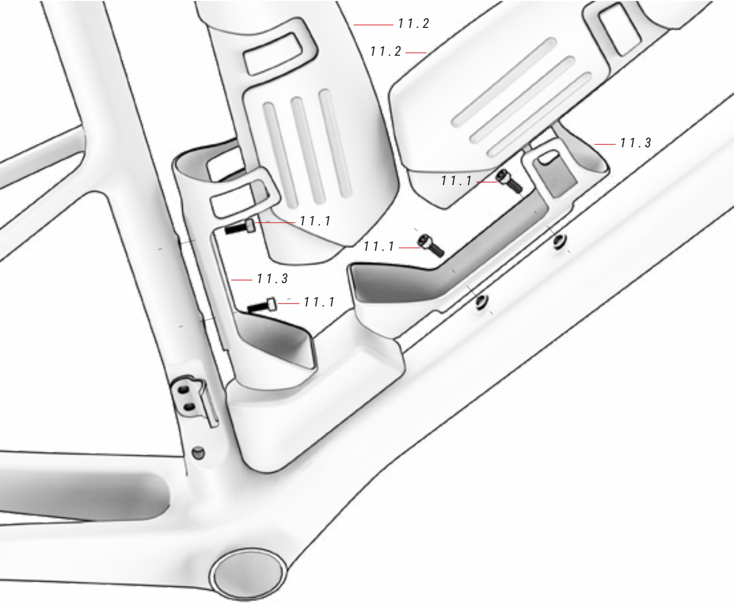
11 SUPORTE GARRAFA
