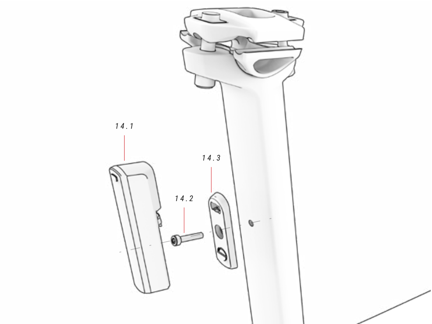
14 LUZ TRASERA ref.: 387435700
