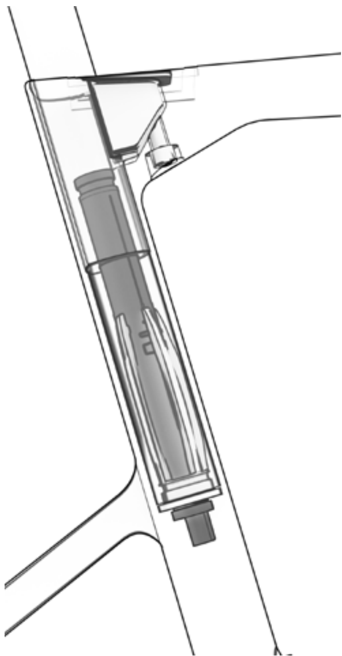
13 SOPORTE DI2 EN TIJA ref.: 387458500
