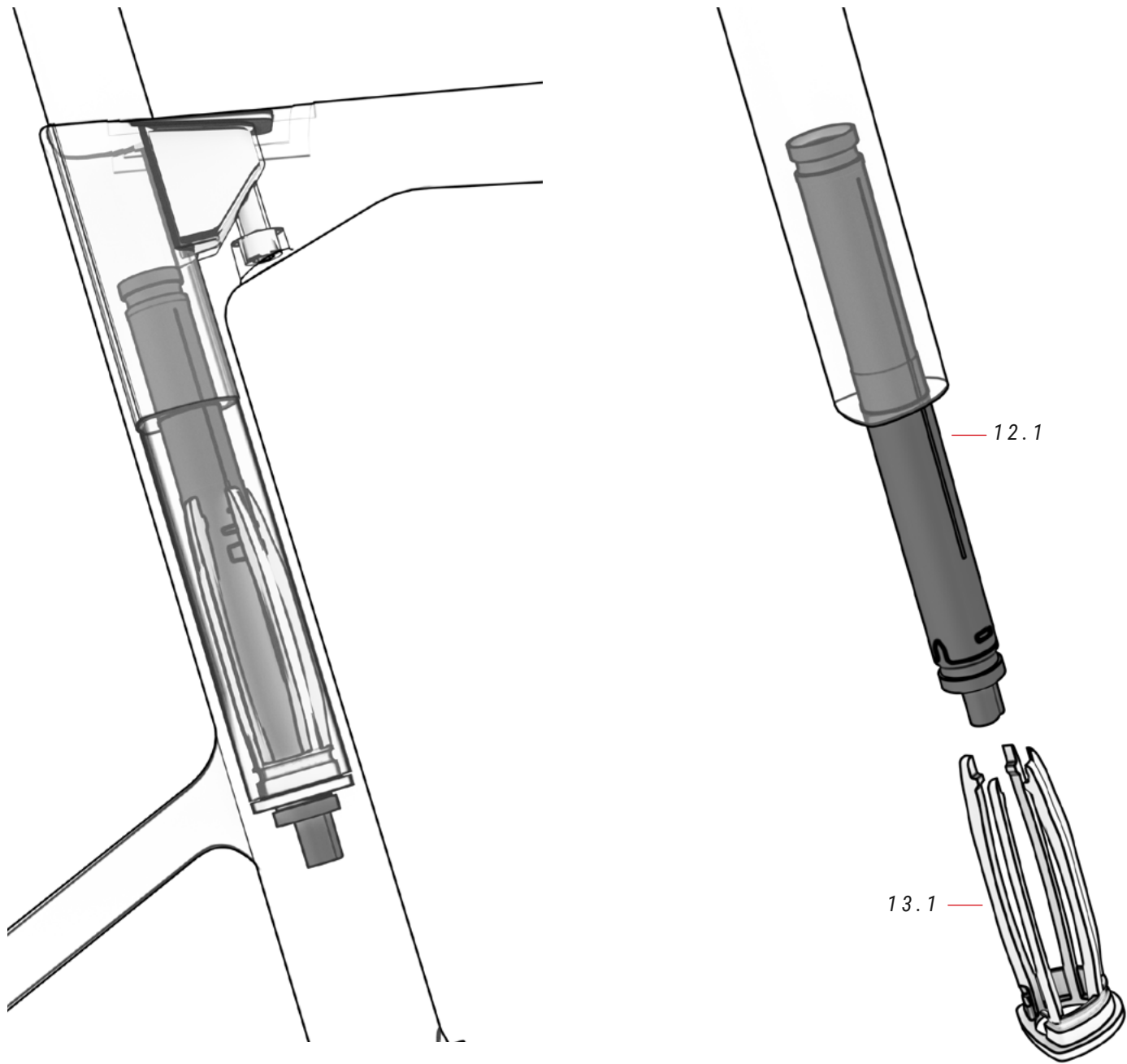
13 SOPORTE DI2 EN TIJA ref.: 387458500
